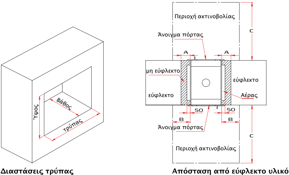
Διαστάσεις τρύπας
