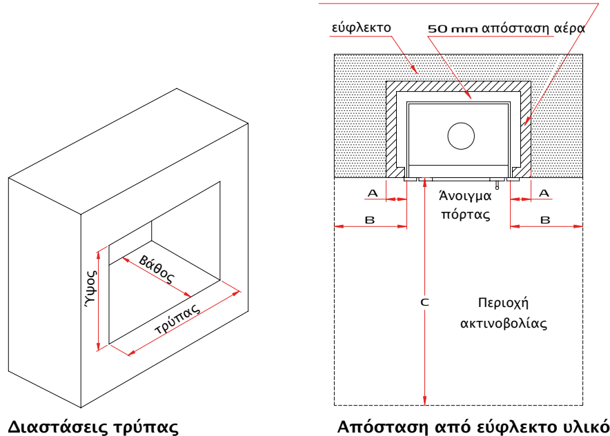
Διαστάσεις τρύπας
