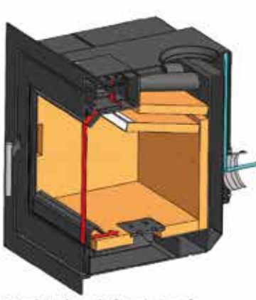
Εισαγωγή αέρα με Airbox στο πίσω μέρος - Προαιρετικό
